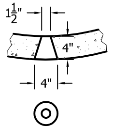
KNOCKOUTS (16 PER ROW)
