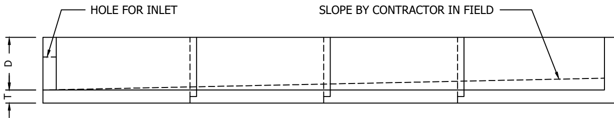
SECTION A-A 1" = 1'-0"
