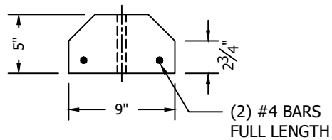
SECTION A-A 1" = 1'-0"
